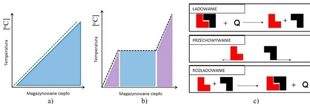
Rys. 3. Metody magazynowania ciepła a) magazyny ciepła jawnego, b) magazyny ciepła utajonego – materiały zmiennofazowe, c) reakcje termochemiczne (De Garcia i Cabeza 2015)
